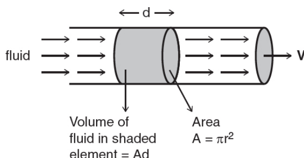
图 6.1 流过一根管子的流体的通量。这里流体的速度（由箭头表示）是恒定的。它的方向垂直于（或者说“正交于”）管子末端所示的那个表面，所以在这种情况下，全部的水都流过那个表面。我在中间特意标出的那一小段圆柱形流体，体积为 V = Ad ，即面积为 A (= \pi r^2) 的圆形底面乘以长度 d 。于是，流体以 A \frac{d}{t} 的速率（单位时间的体积）流过管子末端的阴影表面。但 \frac{d}{t} 是距离 / 时间，也就是速率，所以速度向量就是这个速率、沿着所示的方向。这意味着，在给定时间内流过管子末端的流体量——即通量——是 Av 。这个公式说得通，因为流动越快、面积越大，在给定时间内穿过管子末端的流体体积（或分子数目）就越多。当管子的出口被部分堵住、或者与流向成一定角度时，情况就更为复杂。举例来说，如果流动方向与它所穿过的表面的（法线）成角度 \theta ，你就需要向量 \mathbf{v} 在那个法线方向上的分量。这是因为通量是流过——也就是穿过——表面的流体量。于是，通量的公式就变成了标量积 \mathbf{A} \cdot \mathbf{v} (= Av \cos \theta) 。把 \mathbf{A} 做成向量，意味着要规定：一个曲面的方向被定义为它的法线方向。然而，当你的表面是弯曲的或形状不规则时，你就需要用向量微积分来求面积。这时通量的一般公式是 \int_s \mathbf{v} \cdot d\mathbf{A} 。不过我提这个只是为了完备起见——我们后面不会再用到它。（图内标注为英文： fluid = 流体； Volume of fluid in shaded element = Ad = 阴影部分流体的体积 = Ad ； Area A = \pi r^2 = 面积 A = \pi r^2 。）
