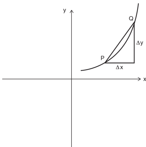
图 2.4 直线 PQ 的斜率是 \frac{\Delta y}{\Delta x} ；它逼近 P 与 Q 之间那段图像的梯度。要说得更专业——也更现代——一些，我们需要极限：为了得到 P 处的精确梯度——并由此求出 P 处的导数——你把点 Q 越来越快地移向 P，直到 \Delta x 与 \Delta y 都变成无穷小。于是图像在 P 处的导数，就是当 \Delta x \rightarrow 0 时 \frac{\Delta y}{\Delta x} 的极限。取了极限之后，莱布尼茨的记号 \frac{dy}{dx} 就取代了 \frac{\Delta y}{\Delta x} 。如果你拿到的是一幅距离 x 对时间 t （而不是如图所示的 y 对 x ）的图像，那么梯度——这时是 \frac{dx}{dt} ——就代表速率 v ——即单位时间内的距离。
