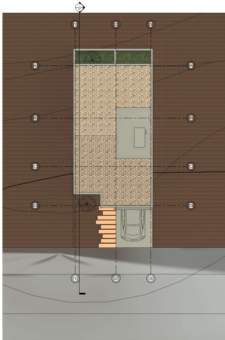
1 IMPLANTACIÓN 1 : 50
