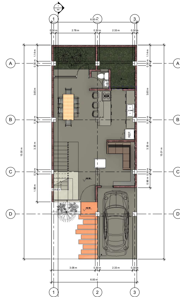
2 PLANTA BAJA 1 : 50
