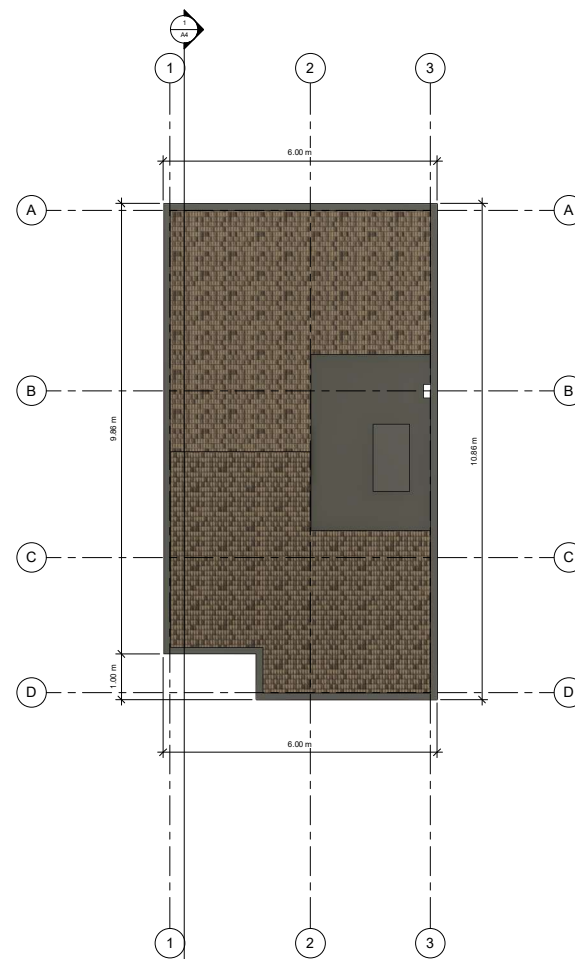
2 CUBIERTA 1 : 50
