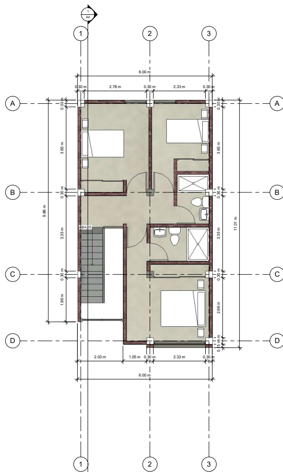
1 PLANTA ALTA 1 : 50
