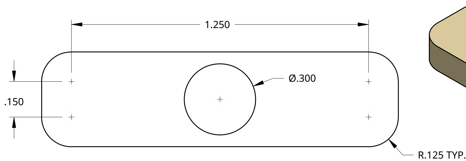
DOUBLE TAB
