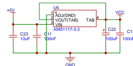
LDO
