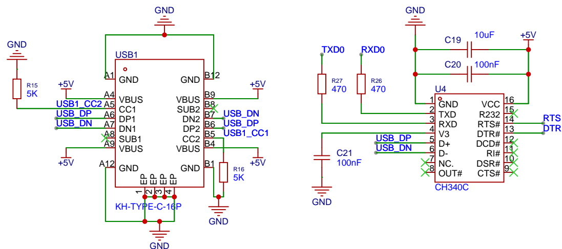
TTL
