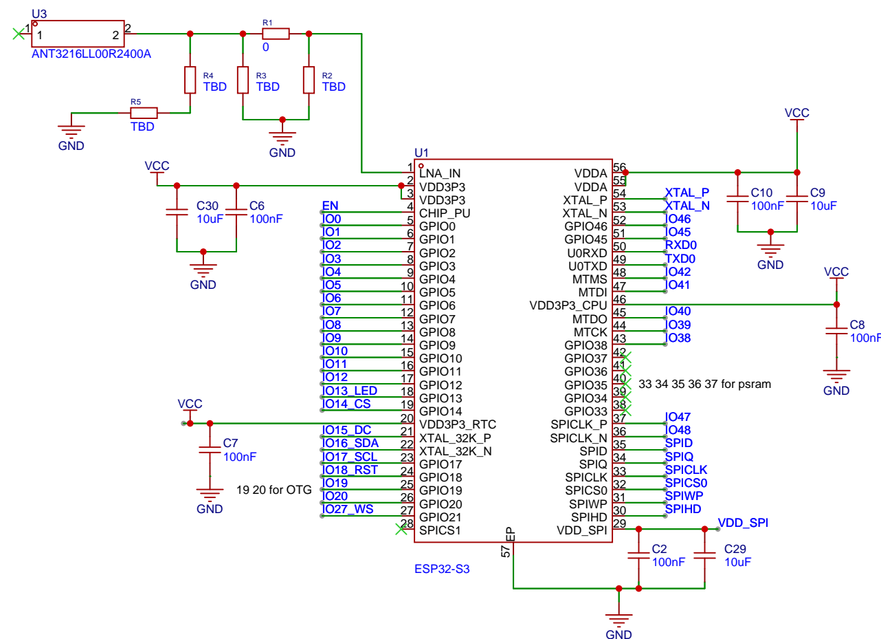
ESP32S3R8
