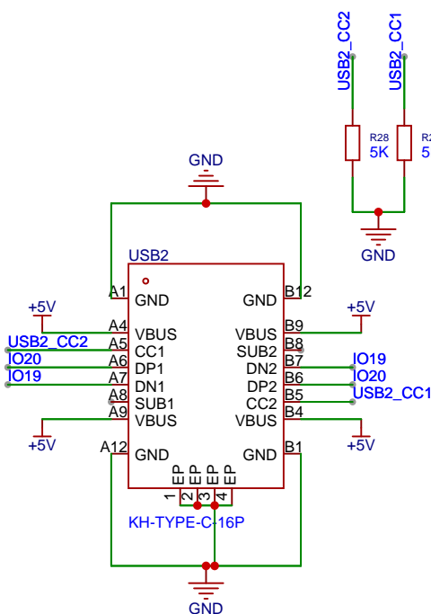
OTG
