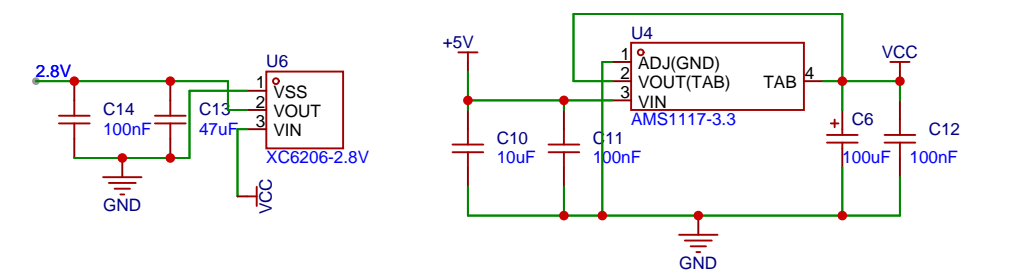
LDO
