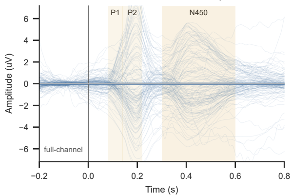
A SuS full-channel butterfly
