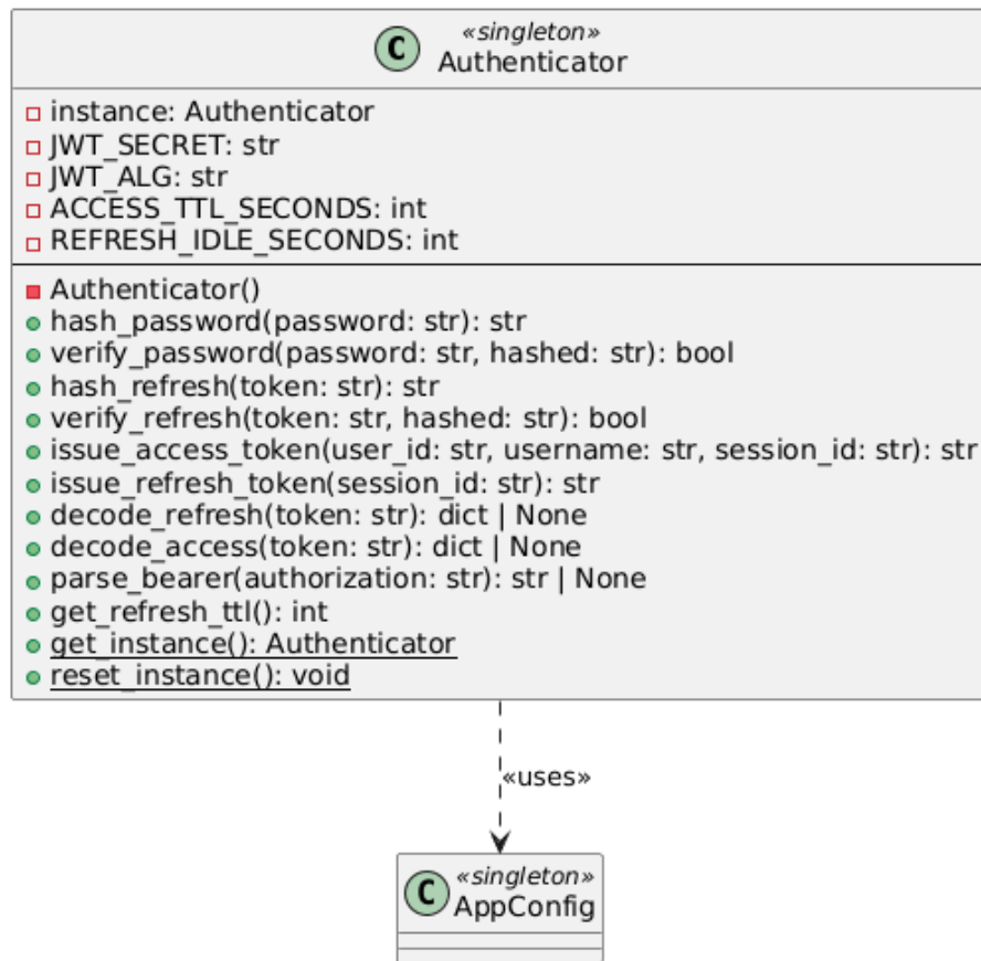
3.12. ábra. Az Authenticator osztály
