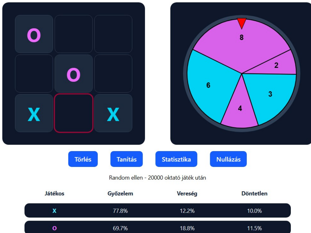
2.22. ábra. MENACE játékszimulációs-panel
