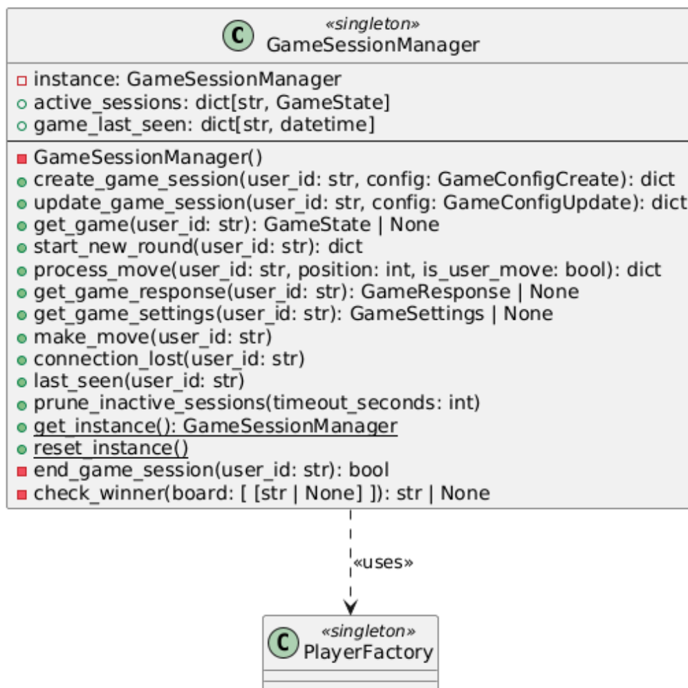
3.13. ábra. A GameSessionManager osztály
