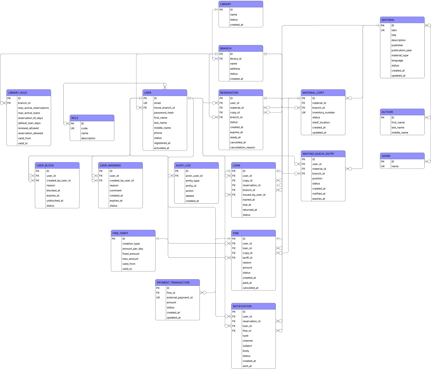
Рис. 2: ER-диаграмма базы данных Library Service
