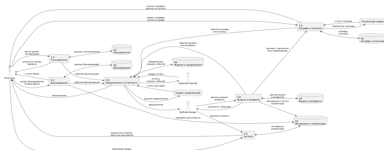
Рис. 1: DFD-диаграмма верхнего уровня для Library Service
