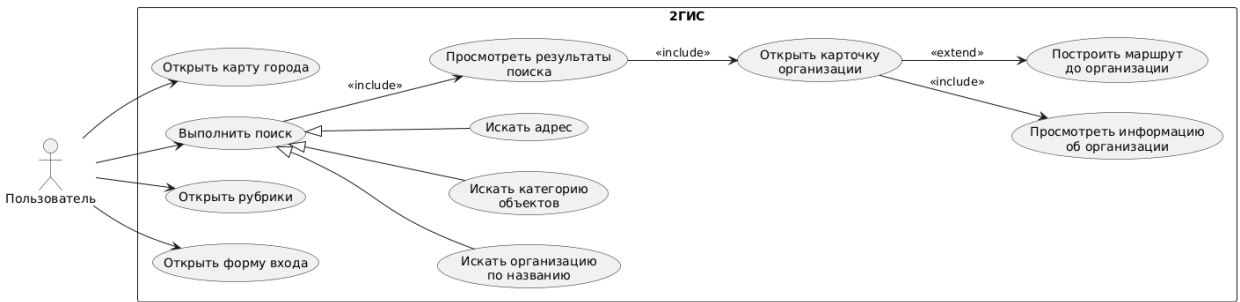
Рис. 2. UseCase диаграмма.
