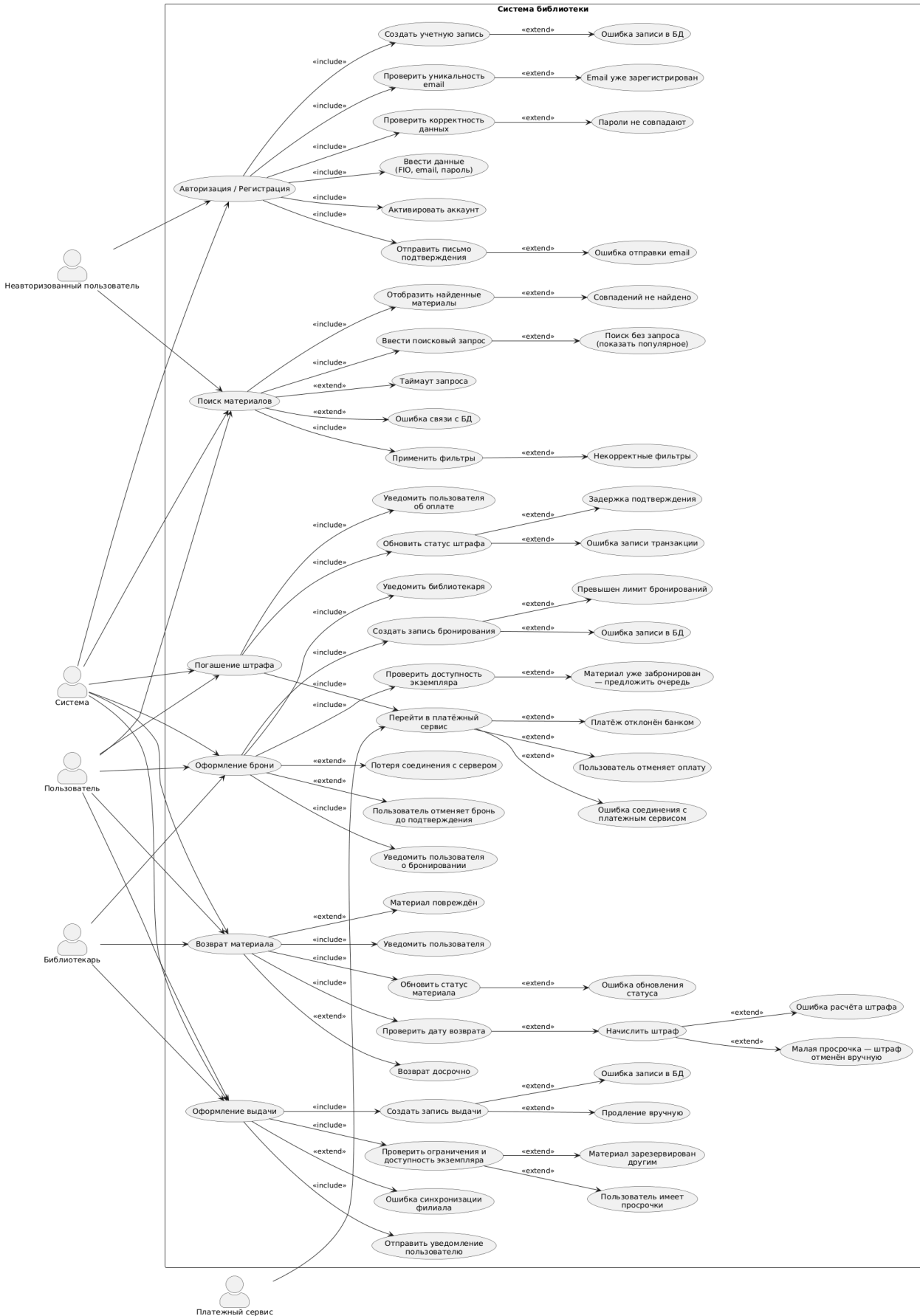
Рис. 1: Use Case-диаграмма для библиотечного сервиса.
