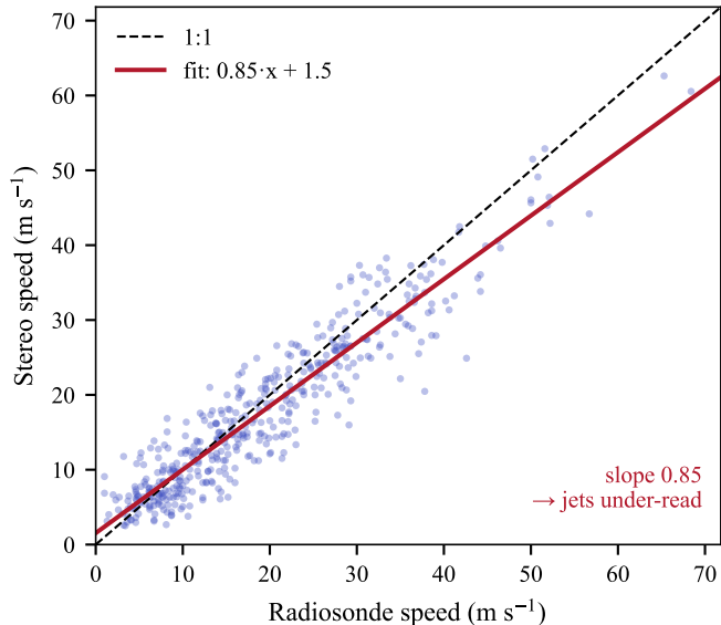
(a) Stereo vs sonde speed (N=454)
