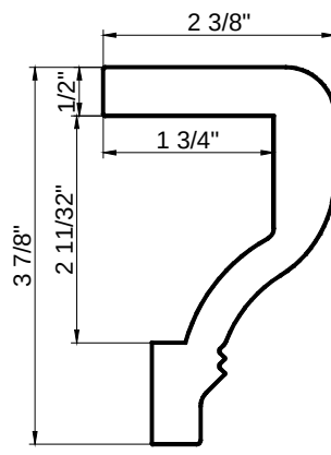
Designer Sill Cap (D)
