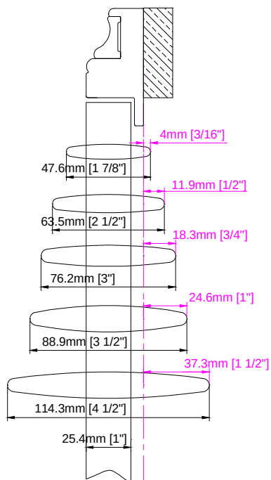
Deco Frame
