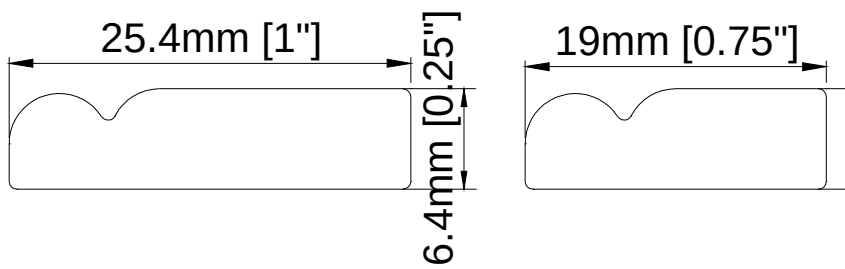
Scribe Trim 1
