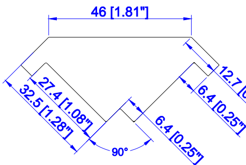
Slim Fit Corner Post for 90 Degree (D)
