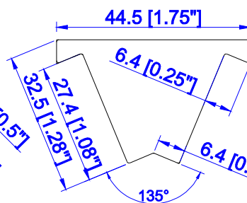
Slim Fit Bay Post for 135 Degree (D)
