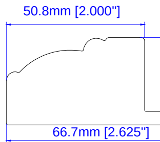
2" Camber Deco Frai
