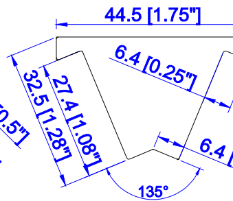
Slim Fit Bay Post for 135 Degree (D)
