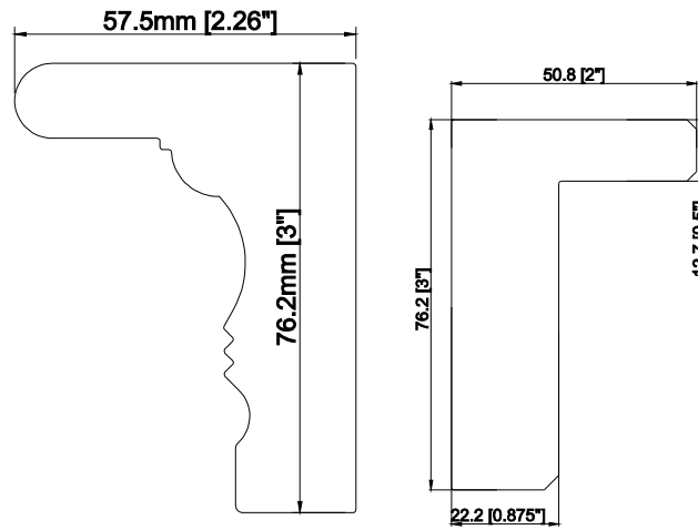
3" Deco Sill Frame
