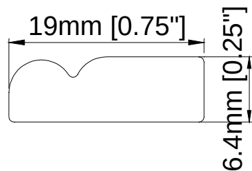
Scribe Trim 2
