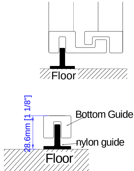
Bottom Guide
