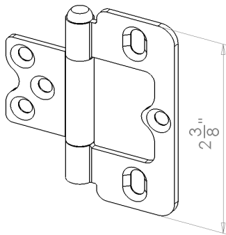
2.375" L Hinge
