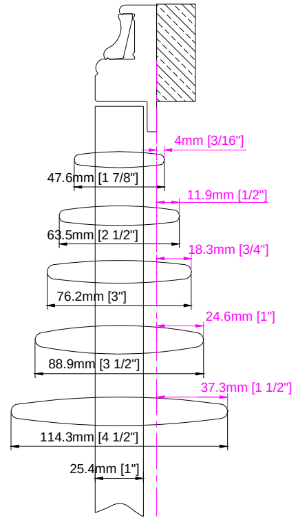
Deco Frame
