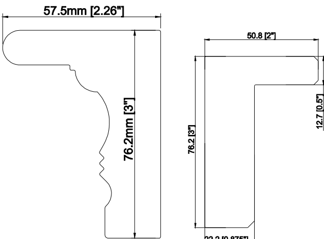
3" Deco Sill Frame
