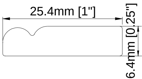
Scribe Trim 1
