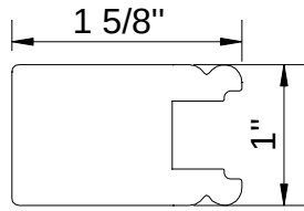
1 5/8" Butt Stile
