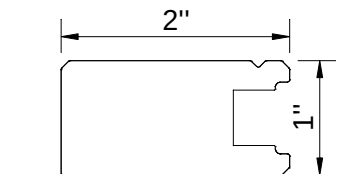
2" Astragal Stile
