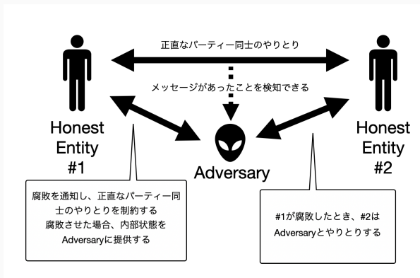
Figure 1: 敵対者とエンティティの関係。敵対者は誠実なエンティティのメッセージを傍受したり、直接エンティティを制御したりすることで、プロトコルに腐敗したエンティティを導入することができる。 4
