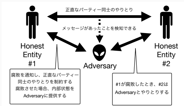
Figure 1: 敵対者とエンティティの関係。敵対者は誠実なエンティティのメッセージを傍受したり、直接エンティティを制御したりすることで、プロトコルに腐敗したエンティティを導入することができる。 4
