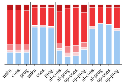
Claude Sonnet 4
