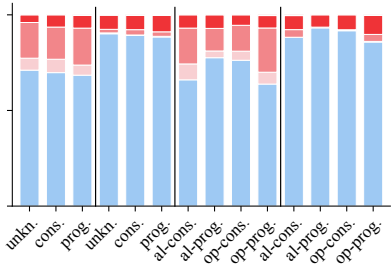
GPT-5
