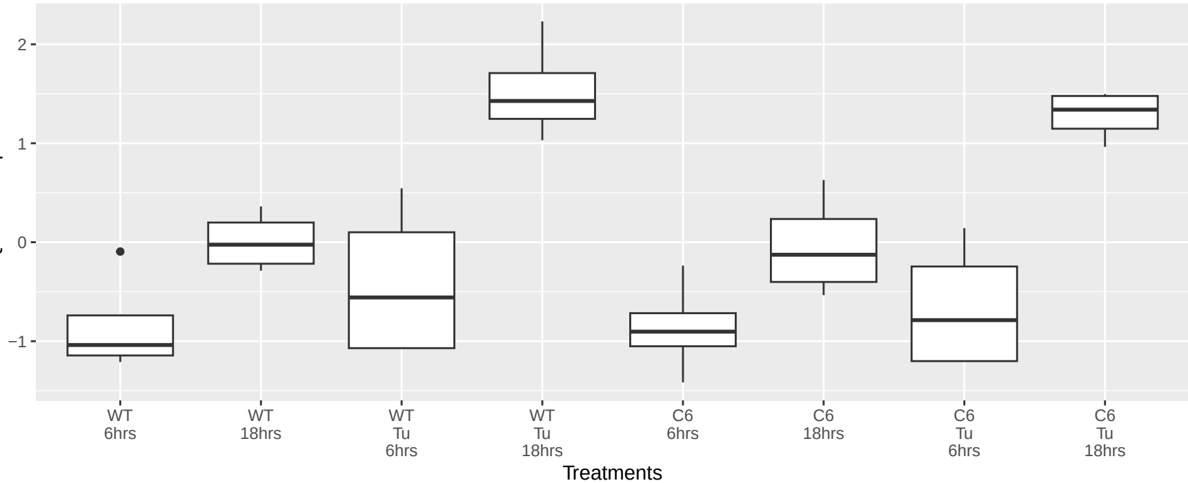
FRG1.Q14331 Expression
