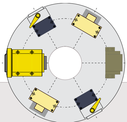
Équipement D 745 – 6 porte-outils répartis régulièrement
