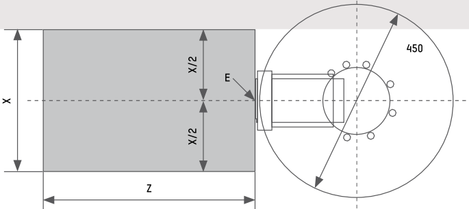
Équipement de la table revolver flexible en fonction de vos besoins
