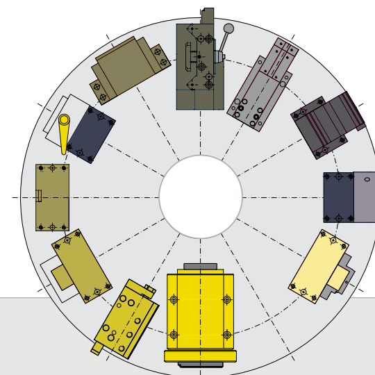
Équipement D 900 – 12 porte-outils répartis régulièrement
