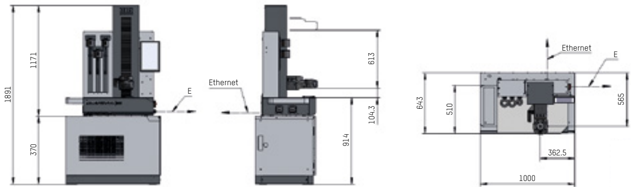
»powerShrink 300«
