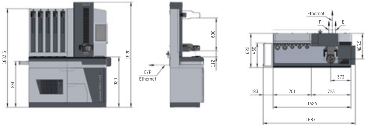
»powerShrink 600«
