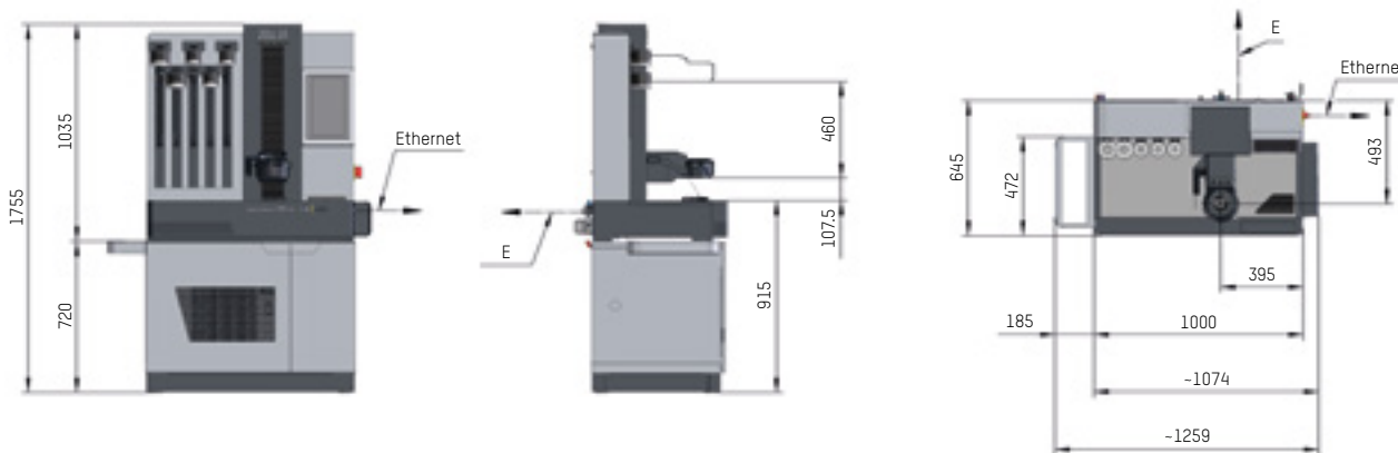
»powerShrink 600«
