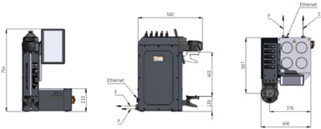
»powerShrink 200«
