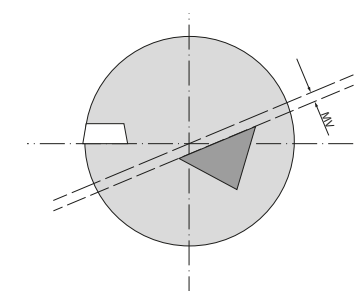
Messung Schneidenüberstand / Mittenversatz (MV) Stirnschneide (Messprogramm 738 am ZOLLER-Universalmessgerät »smartCheck«)
