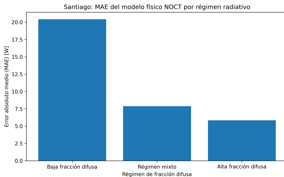
Figura 1: MAE del modelo NOCT por régimen de fracción difusa para la simulación asociada a Santiago.
