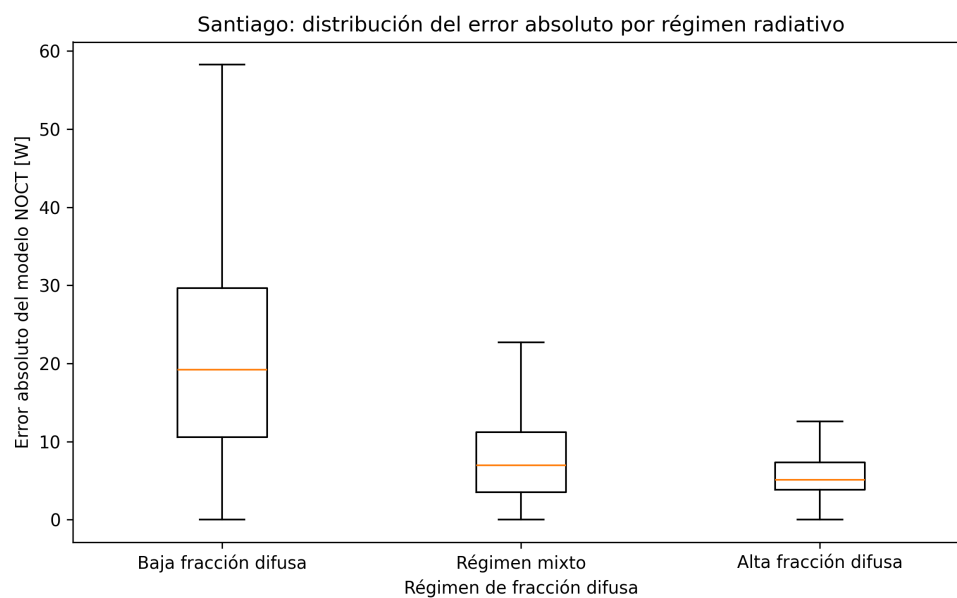
Figura 2: Distribución del error absoluto del modelo NOCT por régimen de fracción difusa; los valores extremos no se muestran en el boxplot.
