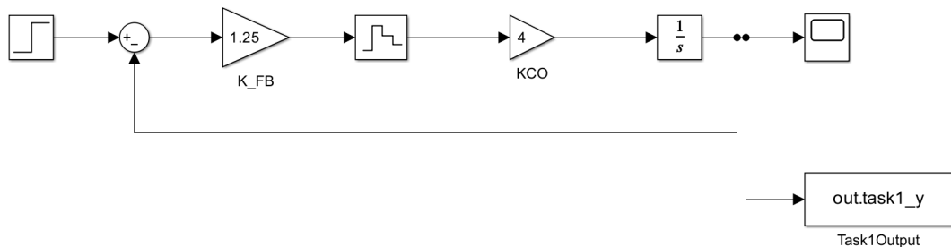
Рис. 1: Схема исследования влияния экстраполятора нулевого порядка
