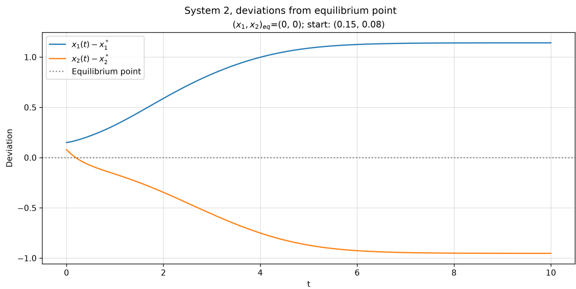
Рис. 8: Переходные процессы системы 2
