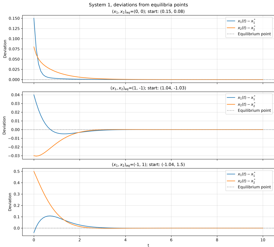
Рис. 7: Отклонения от точек равновесия системы 1
