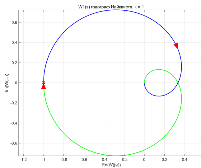
Рисунок 2.2. Годограф Найквиста W_1(s)
