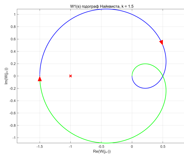
Рисунок 2.3. Годограф Найквиста W_1(s)
