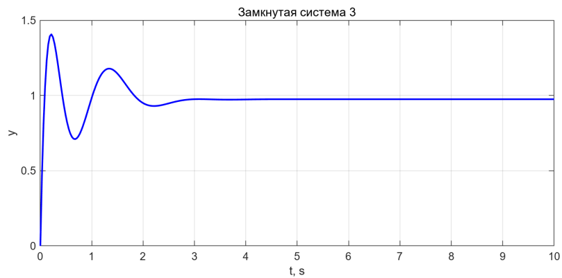
Рисунок 1.6. Переходная характеристика (объект 3)
