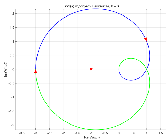
Рисунок 2.4. Годограф Найквиста W_1(s)
