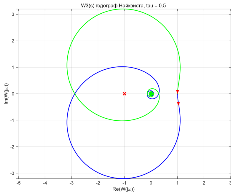
Рисунок 3.3. Годограф Найквиста W_3(s)
