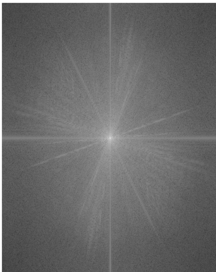
Рисунок 2.2. Логарифм модуля образа
