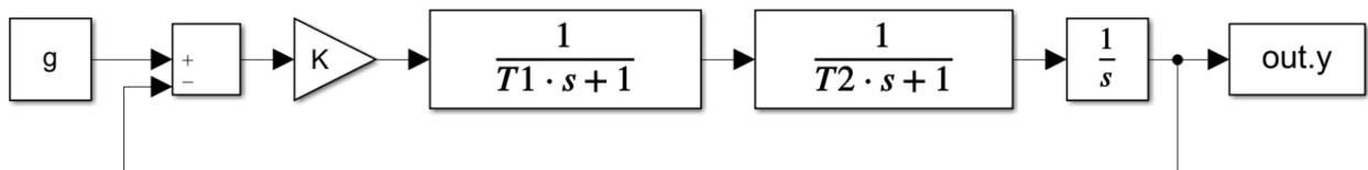
Рисунок 2.1. Схема моделирования
