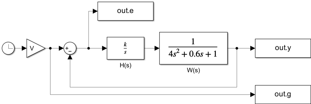
Рисунок 4.4. Структурная схема
