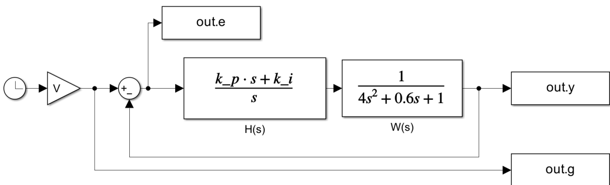
Рисунок 5.1. Структурная схема
