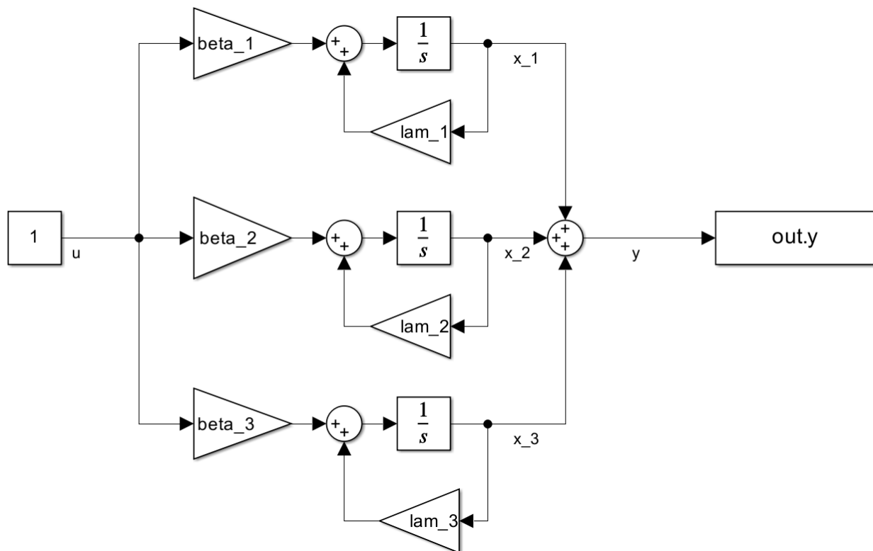
Рисунок 2.4. Структурная схема канонической диагональной формы
