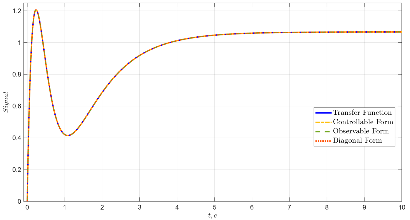
Рисунок 2.6. Графики выходов
