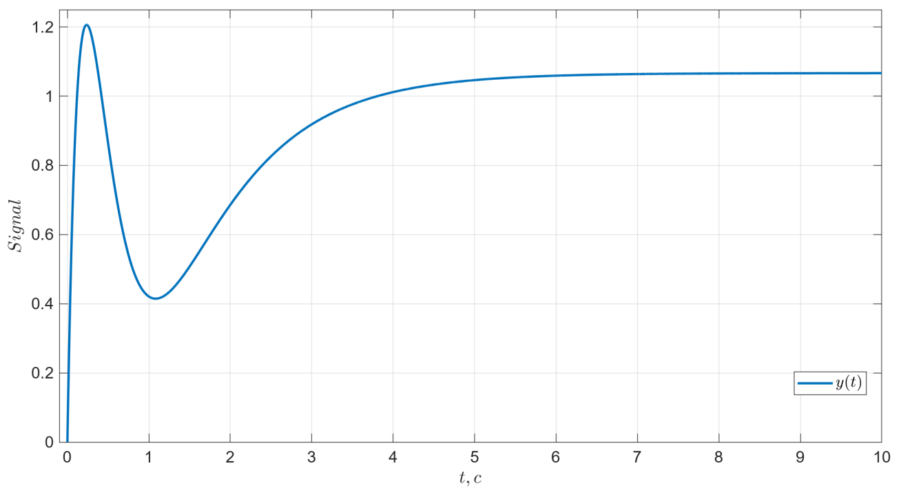
Рисунок 1.3. График выхода
