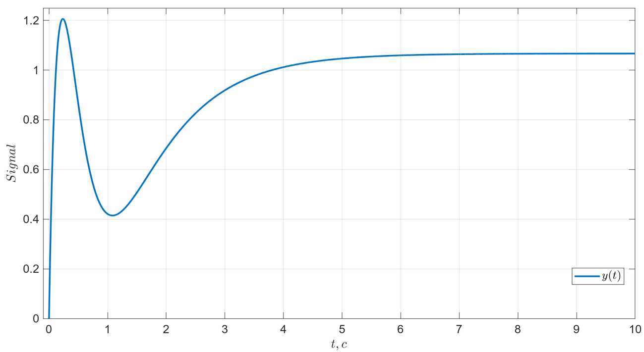
Рисунок 1.3. График выхода
