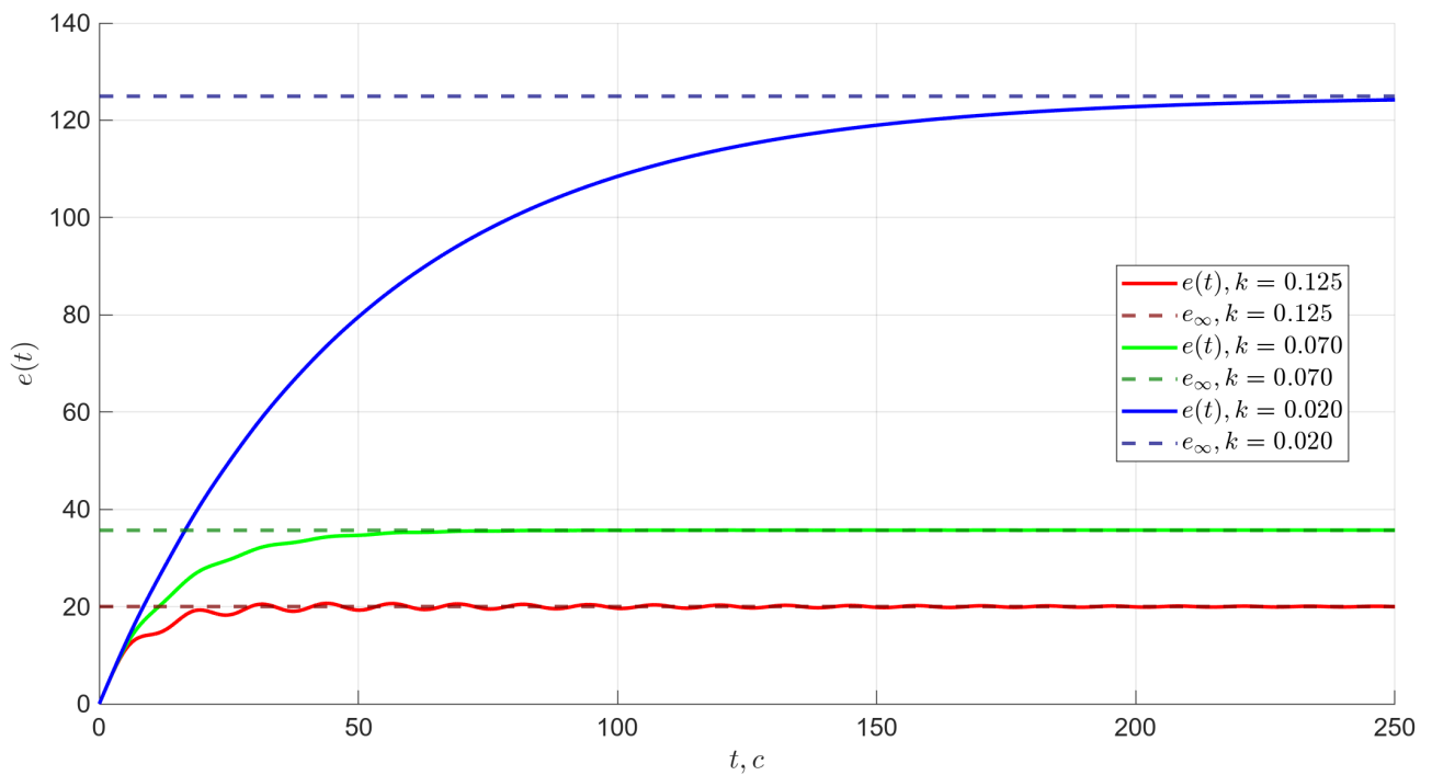
Рисунок 4.6. График ошибки
