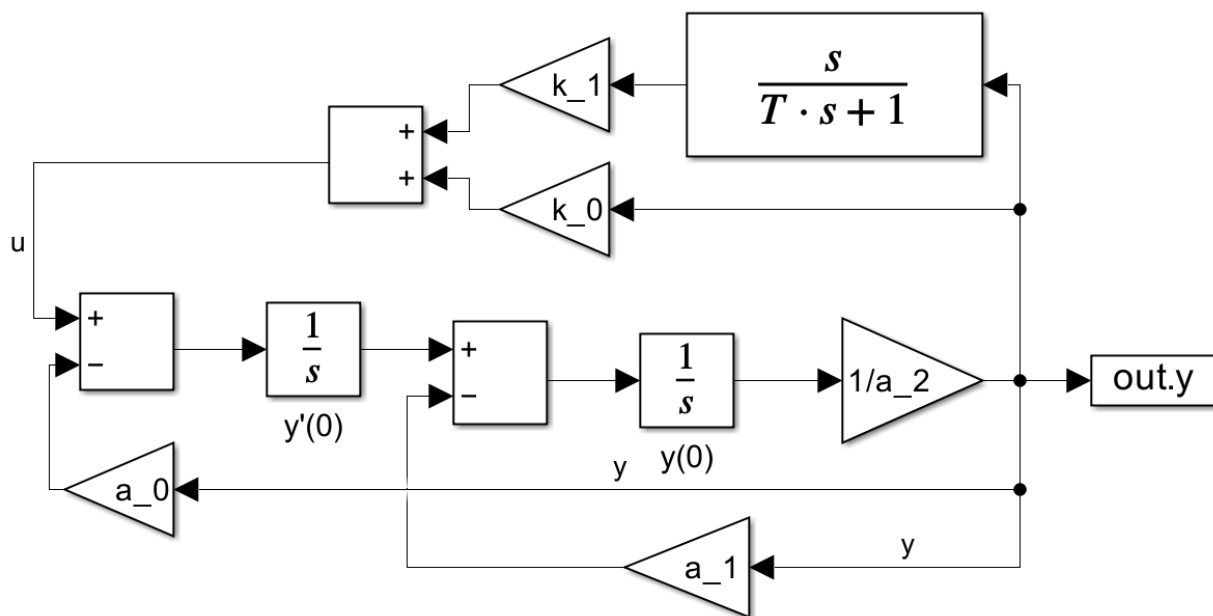
Рисунок 2.1. Структурная схема
