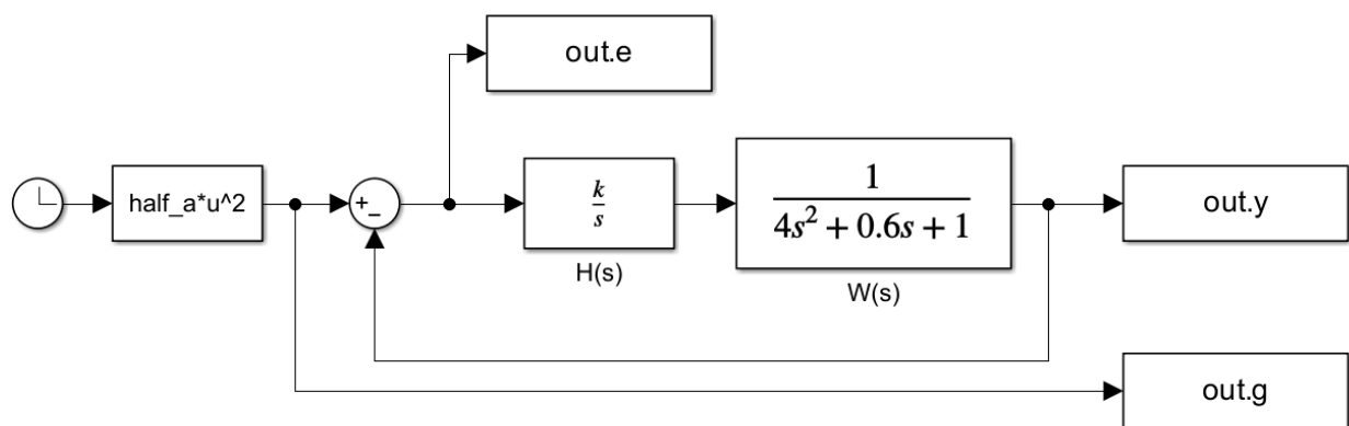
Рисунок 4.7. Структурная схема
