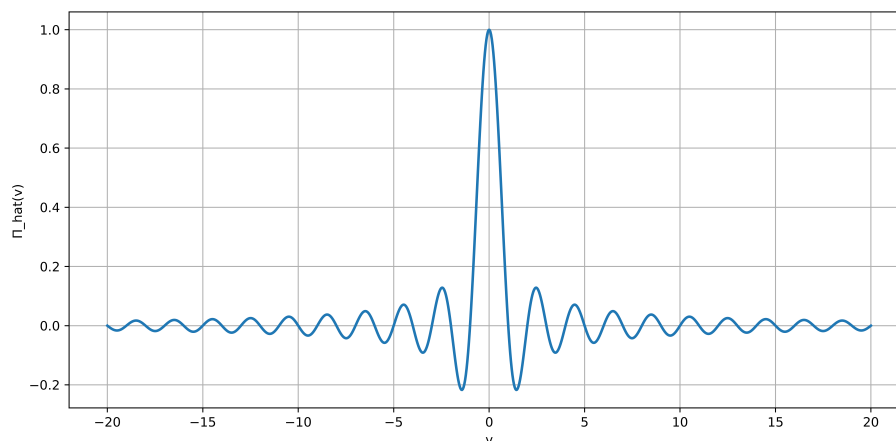
Рисунок 1.2. График \hat{\Pi}(\nu)
