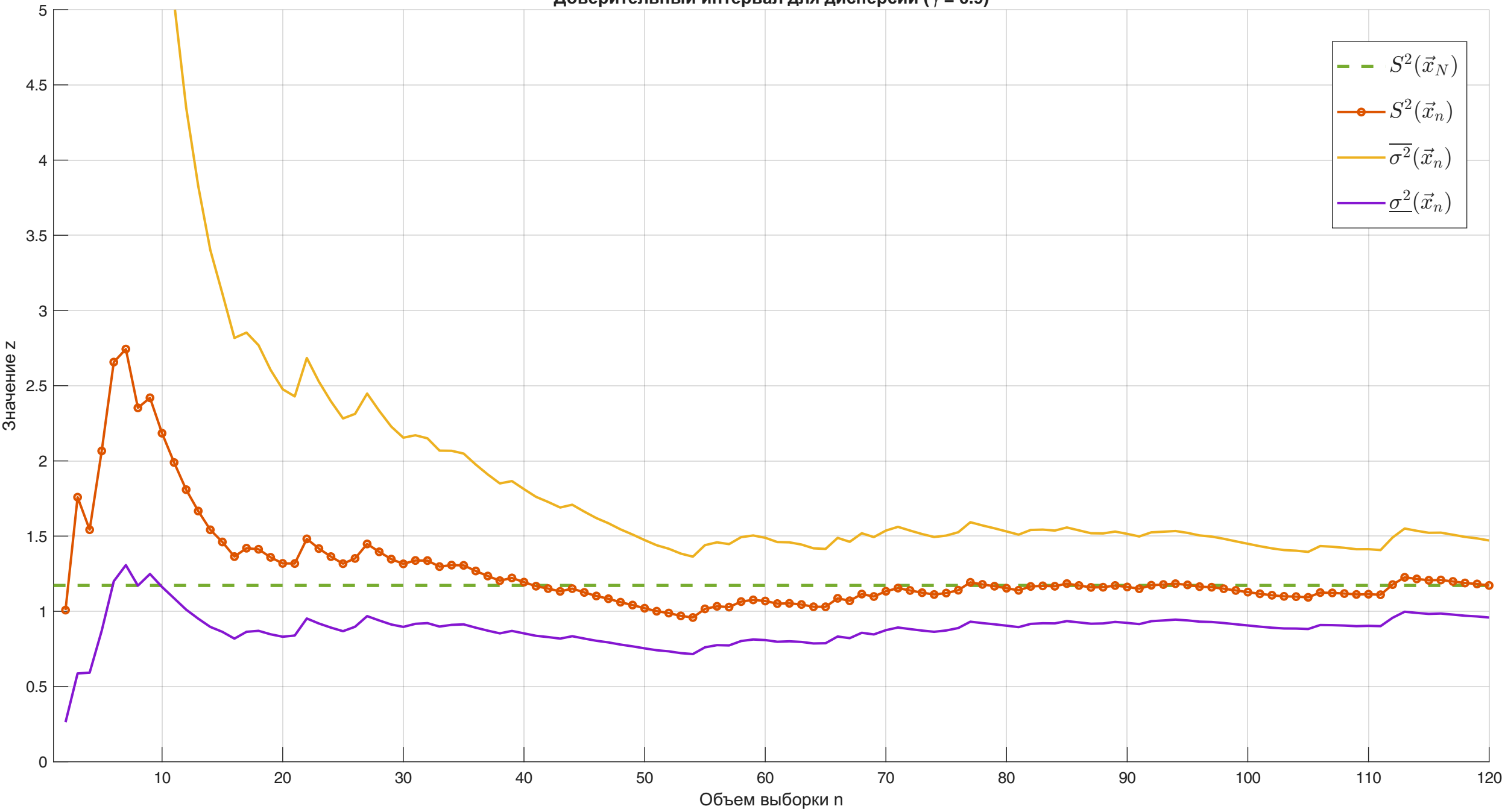
Доверительный интервал для дисперсии ( \gamma = 0.9 )
