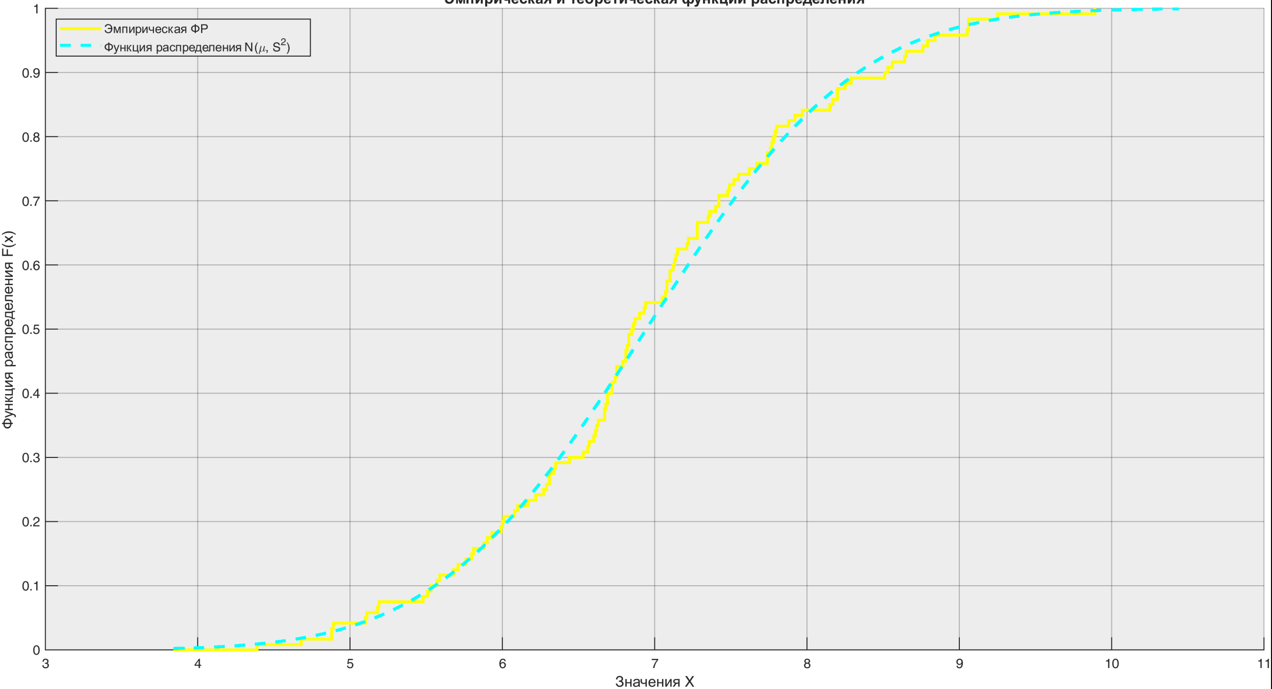
Эмпирическая и теоретическая функции распределения
