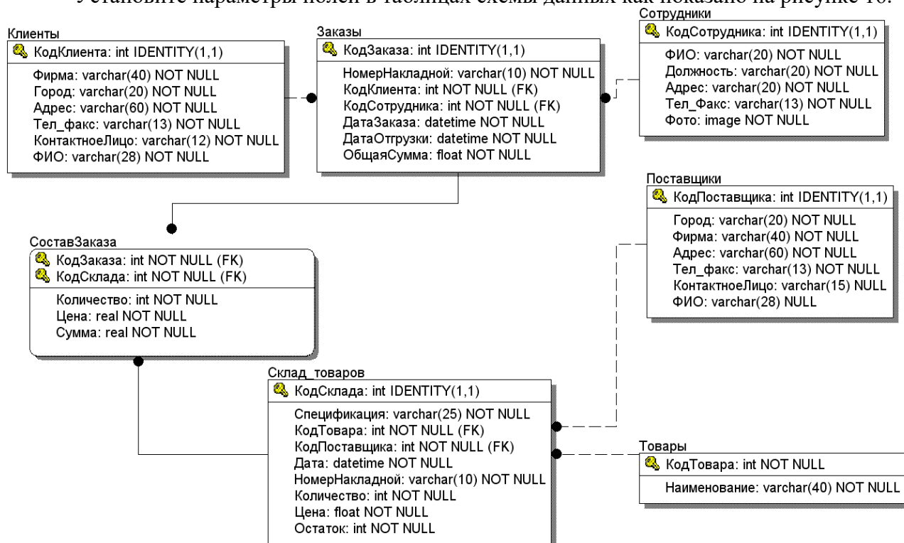
Рис. 16. Окончательная схема базы данных ИС «Заказы»
