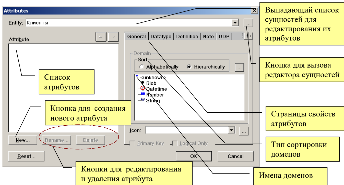
Рис.10. Окно описания атрибутов сущностей
