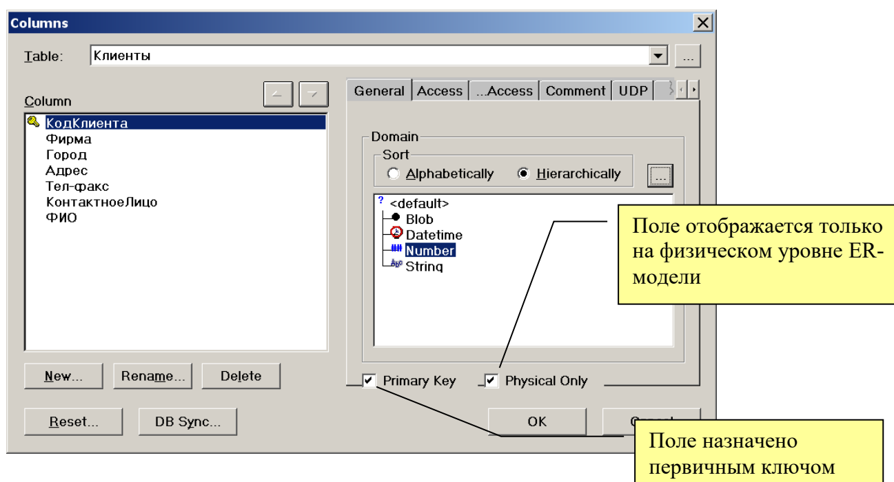
Рис. 12. Описание поля на только физическом уровне таблицы «Клиенты»
