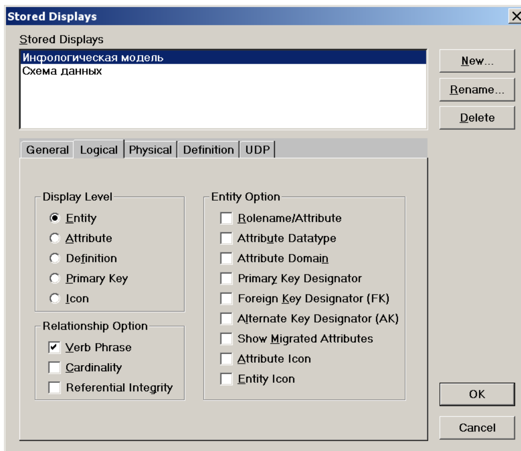
Рис. 3 Окно закладки логического уровня
