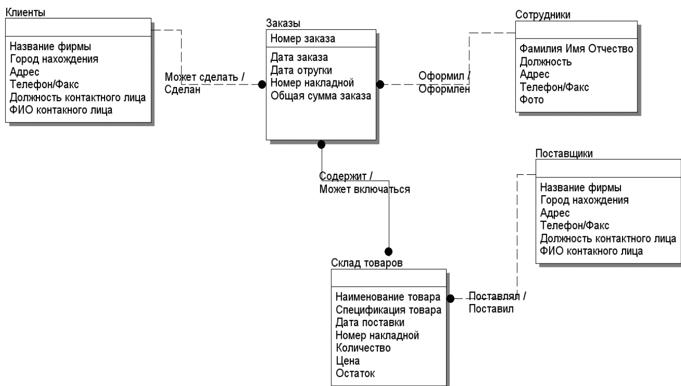
Рис. 11. Инфологическая модель данных ИС «Заказы»
