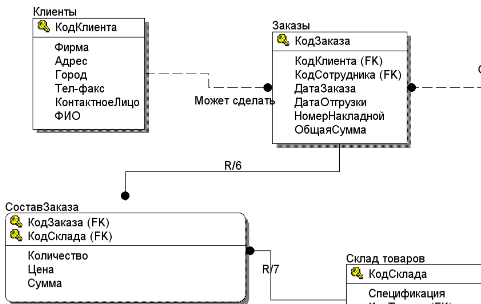
Рис. 14. Замена связей многие-ко-многим промежуточной таблицей «СоставЗаказа»
