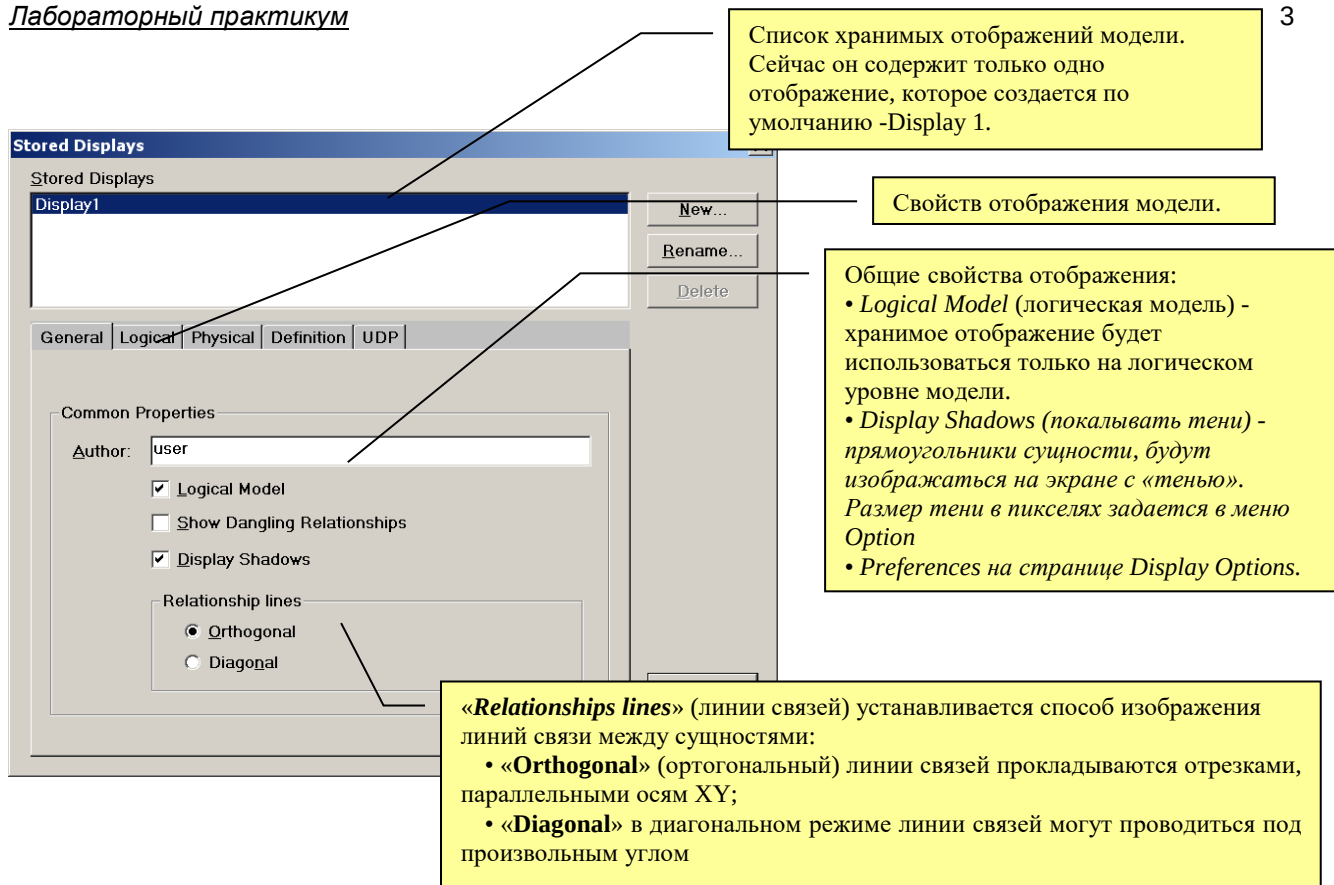
Рис.2 Окно редактора хранимых отображений
