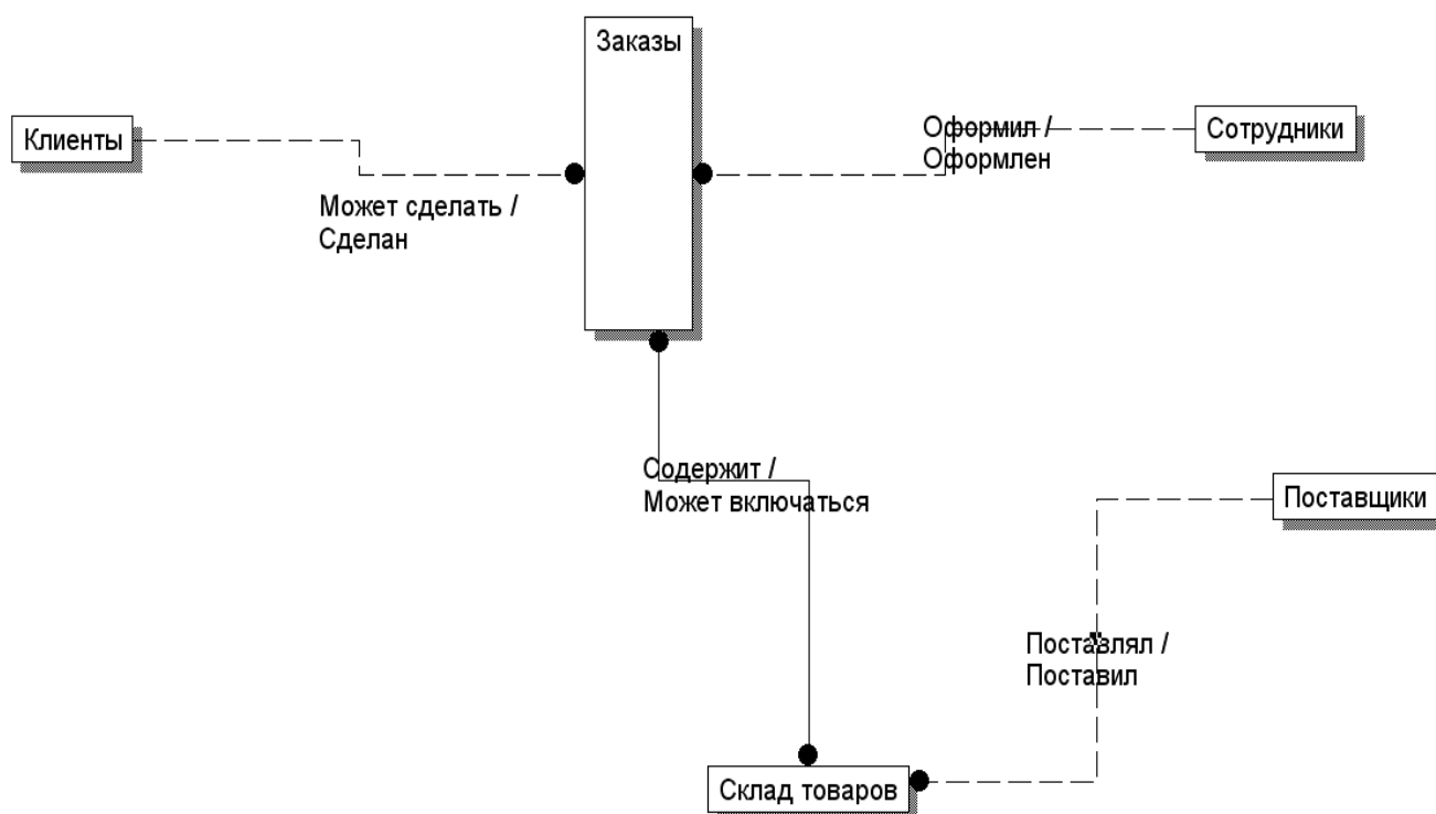
Рис. 9. Инфологическая модель данных ИС «Заказы» на уровне сущностей и связей
