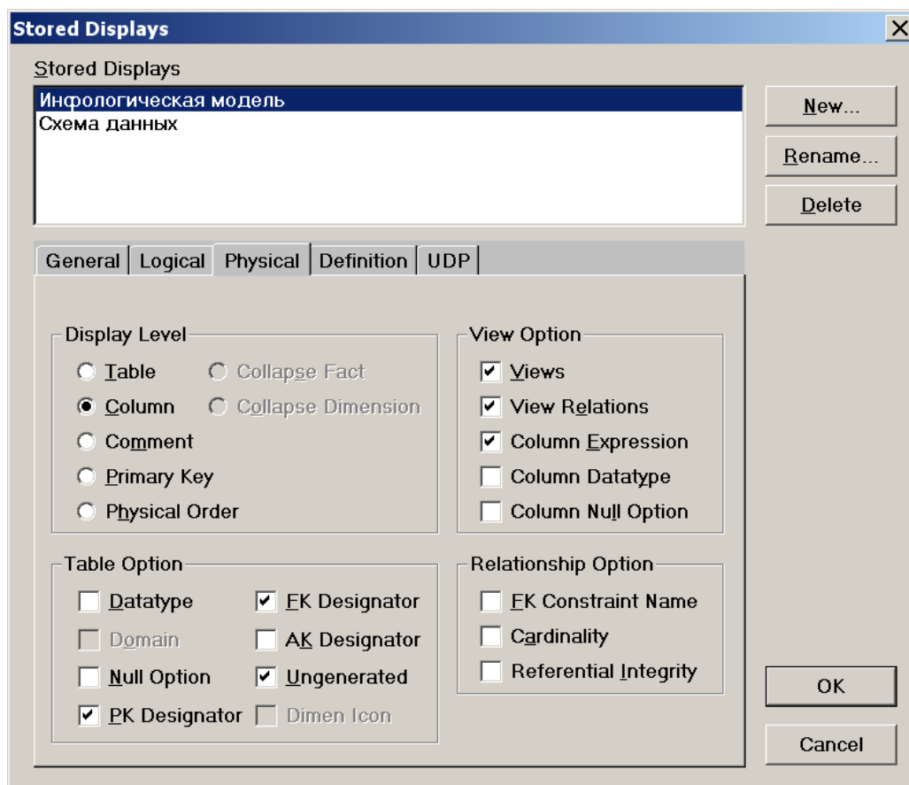
Рис. 4 Окно закладки физического уровня
