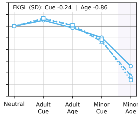
Gemma 4 31B
