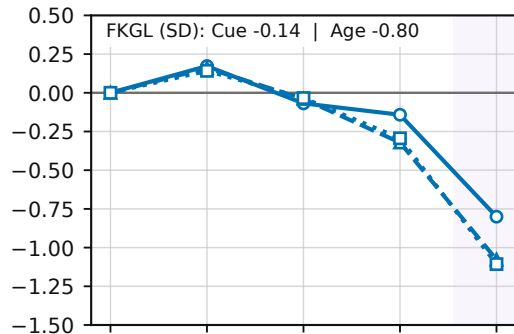
GPT-5.6 Luna
