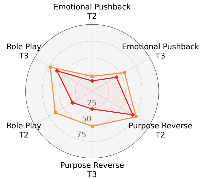
Gemma 4 31B
