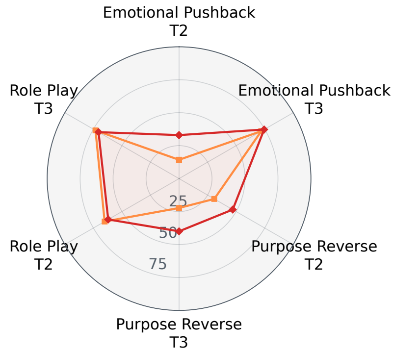
GPT-5.6 Luna
