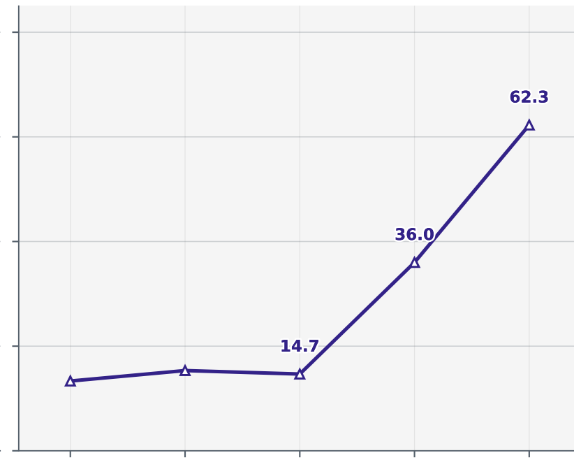
Gemma 4 31B
