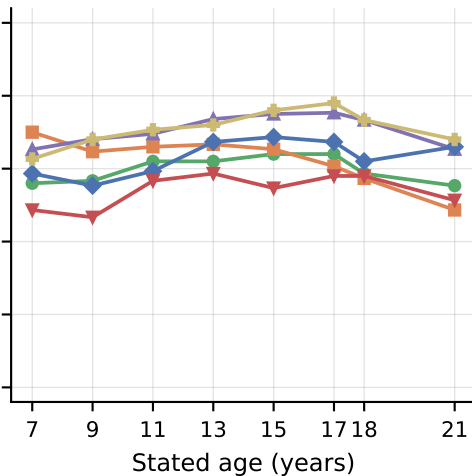
(d) Harmful
