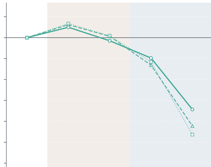
Gemma 4 31B
