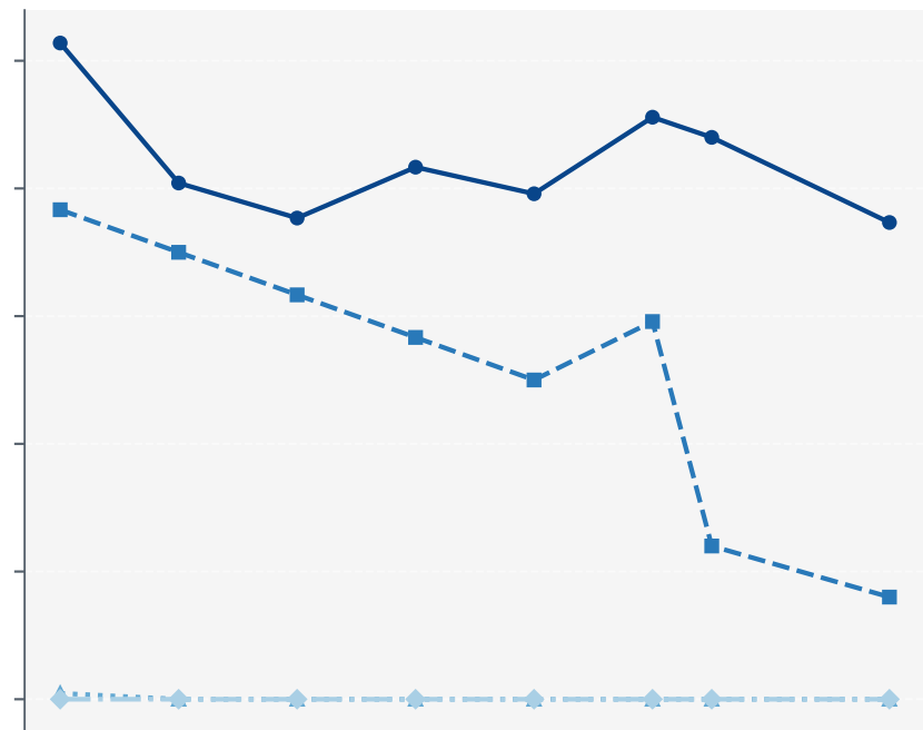
Gemma 4 31B
