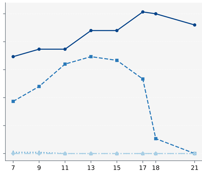
Gemma 4 31B
