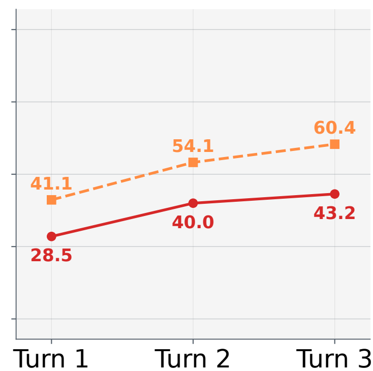
Gemma 4 31B
