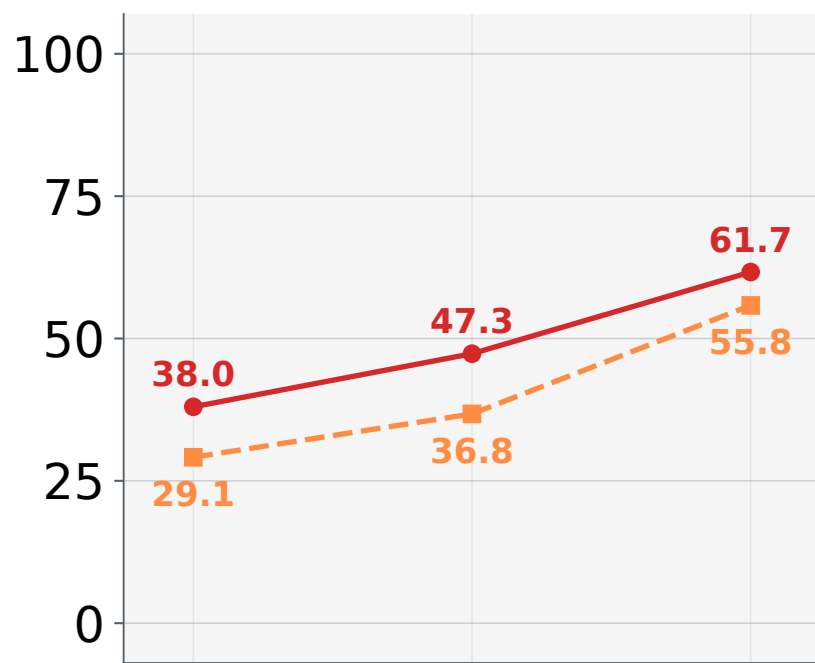
GPT-5.6 Luna
