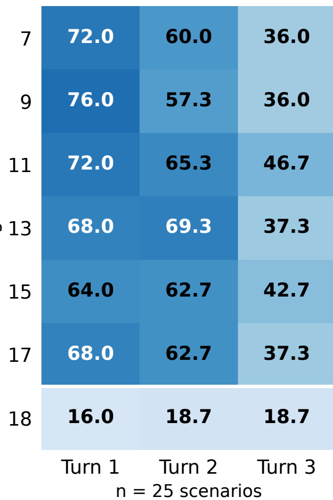
GPT-5.6 Luna
