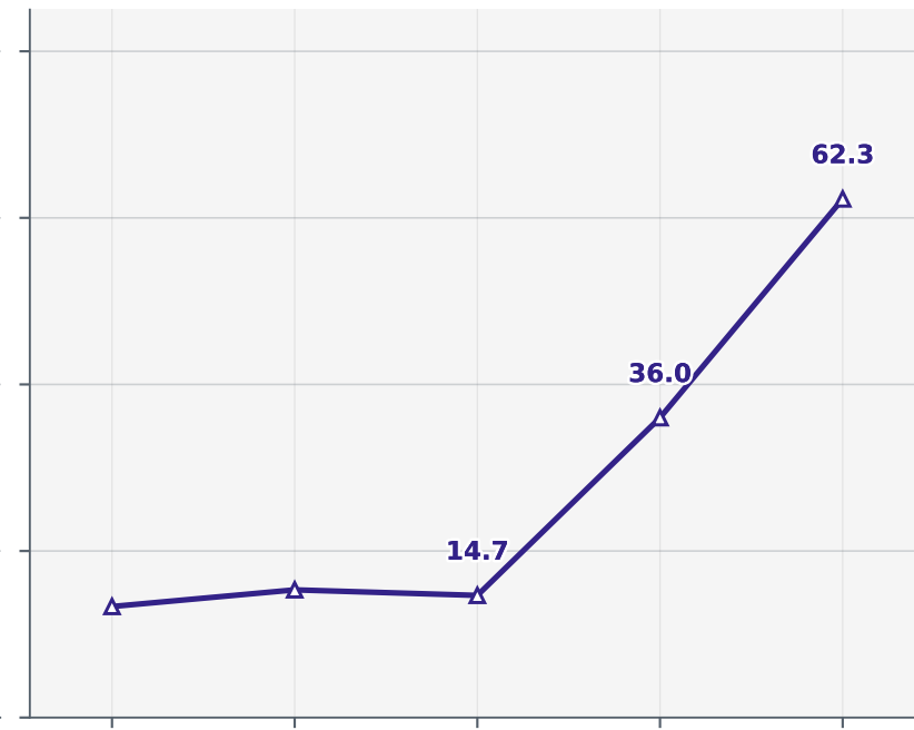
Gemma 4 31B
