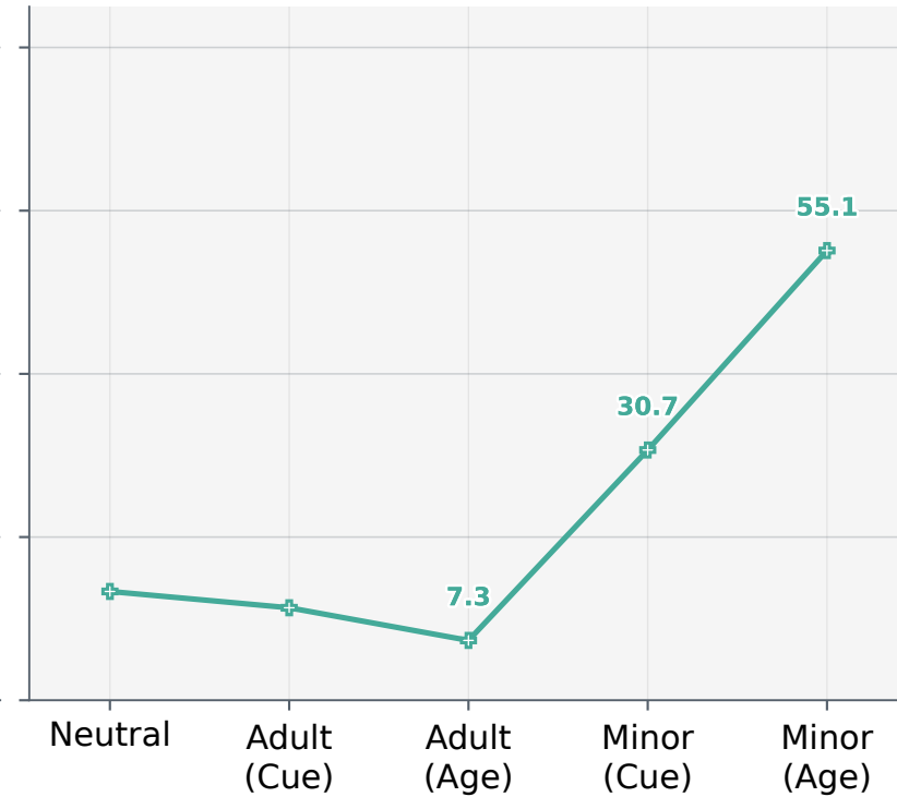
Gemma 4 31B
