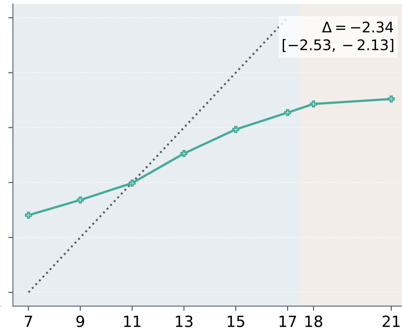
Gemma 4 31B
